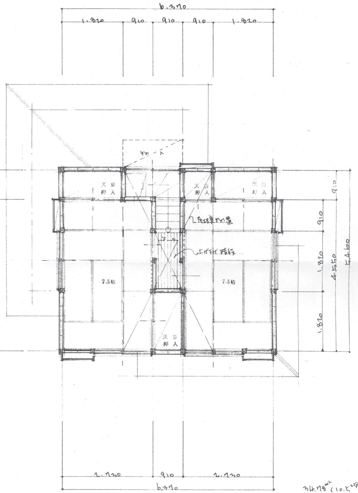
2階平面図 S=1:50
