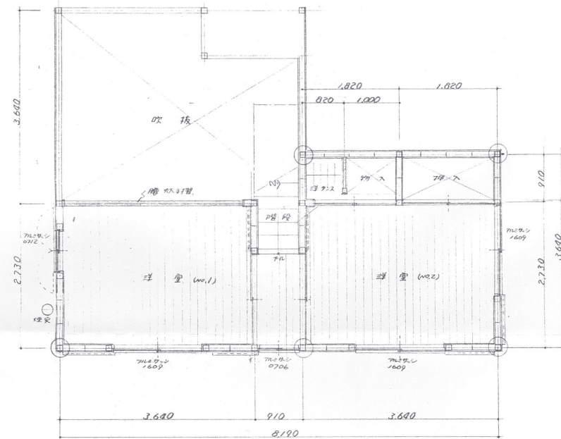
2階平面図
