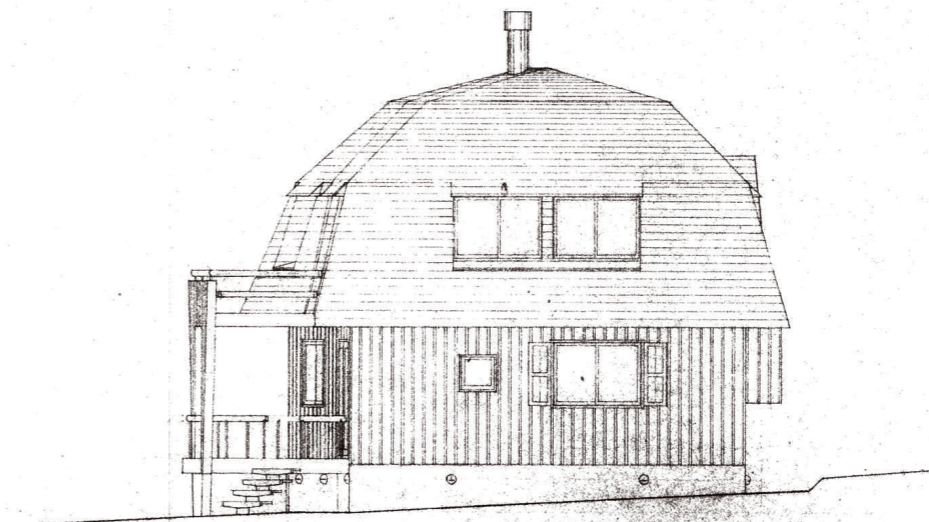
東立面图
