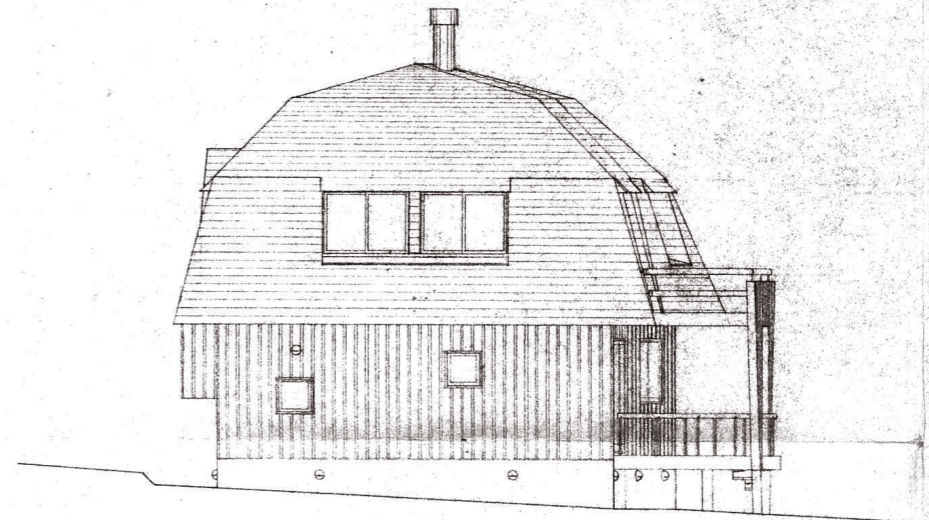
西立面图
