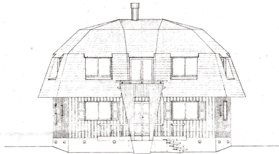
南立面图
